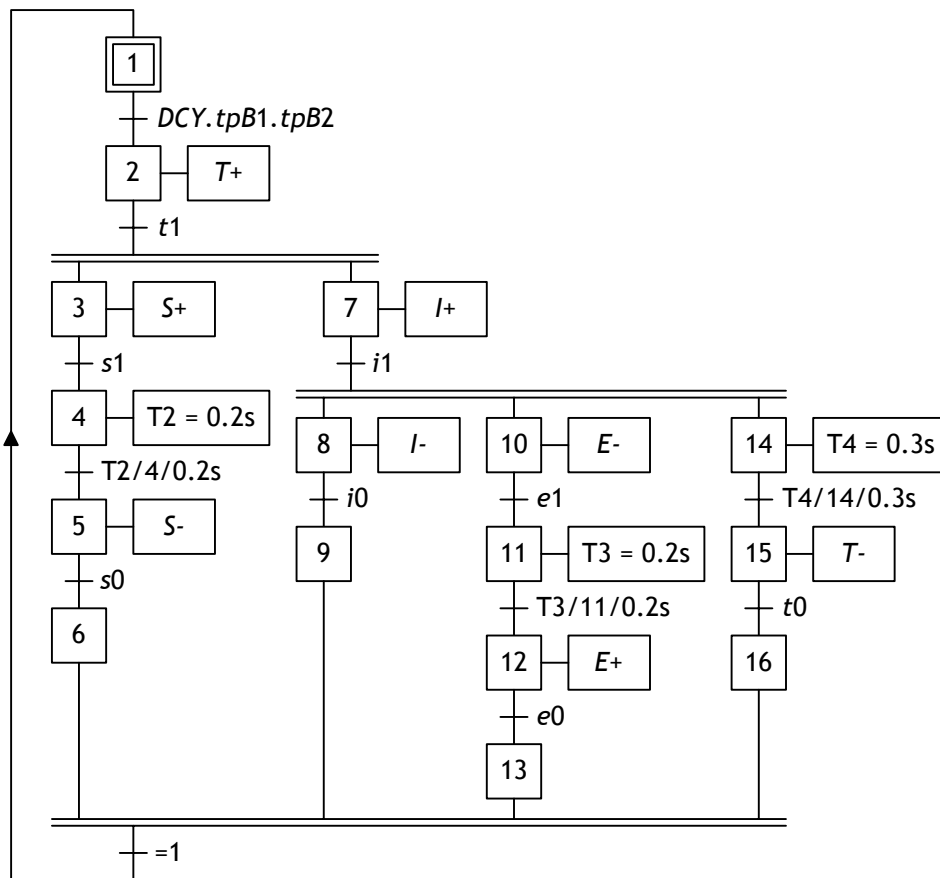
Figure 20 : GRAFCET de niveau 2 du fonctionnement normal du système de sertissage
