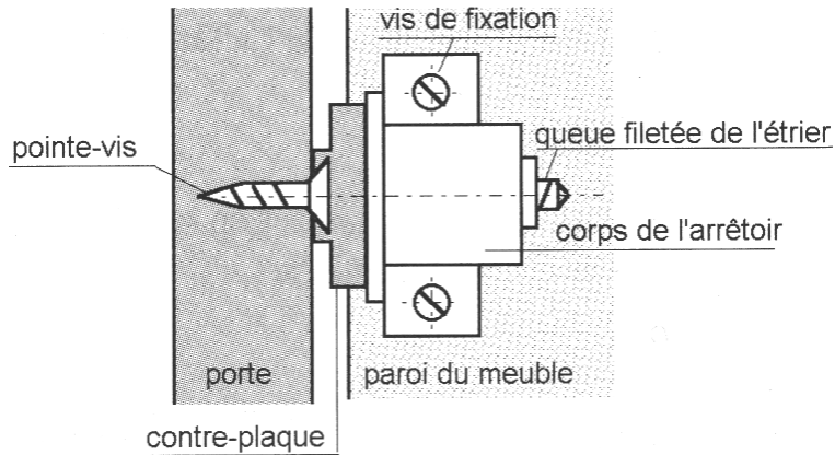
Figure 11 : Fermeture magnétique
