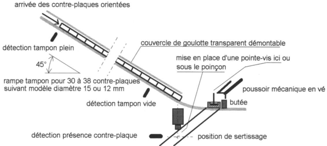
Figure 14 : Glissière et poussoir mécanique
