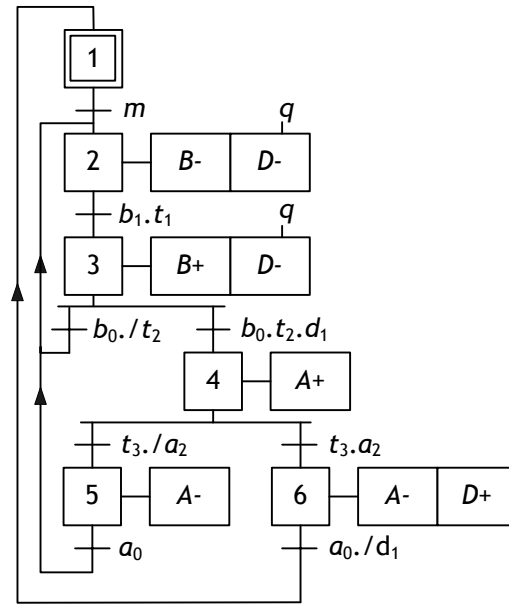
Figure 8 : GRAFCET du fonctionnement normal de la machine d'encaissage semi-automatique
