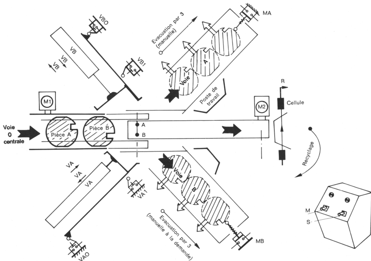
Figure 9 : Système de tri automatique
