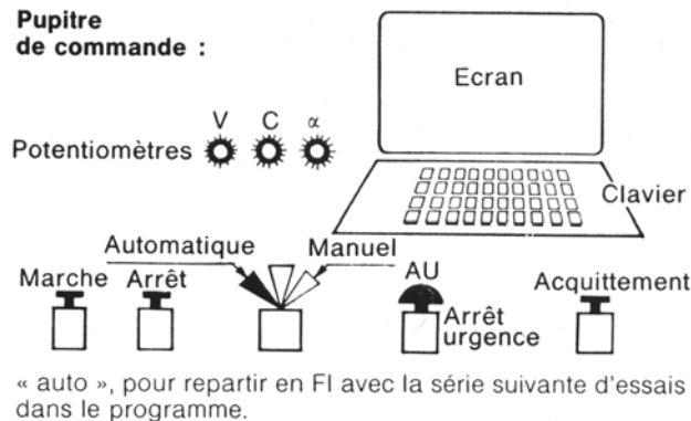
Figure 3 : Pupitre de commande comportant un clavier et un écran
