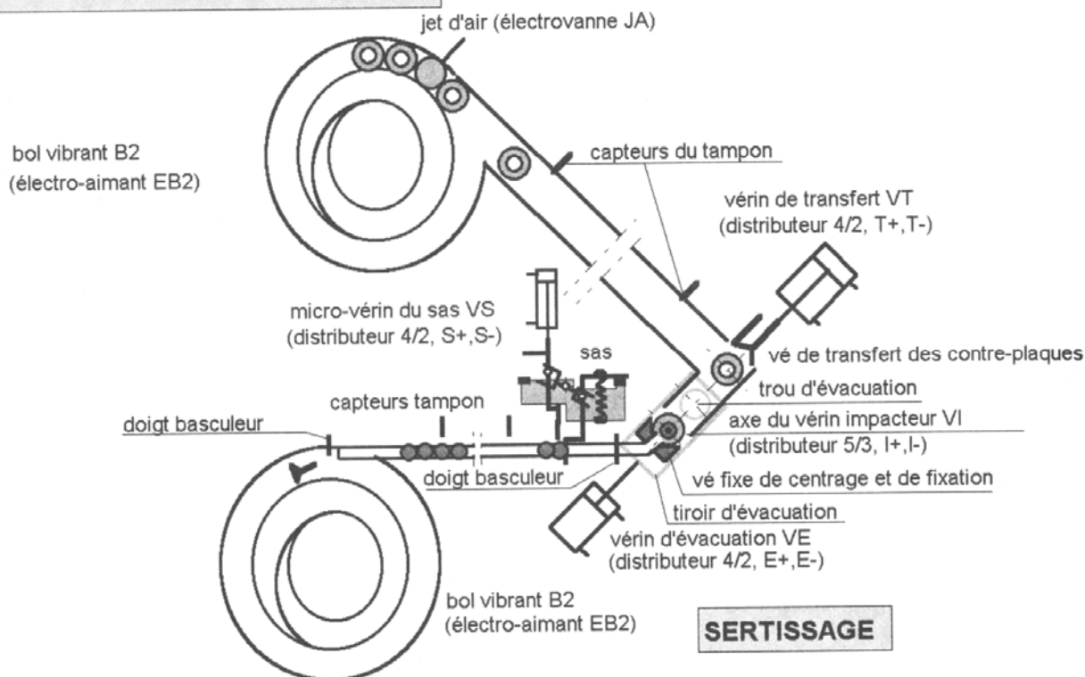
Figure 18 : Machine de sertissage
