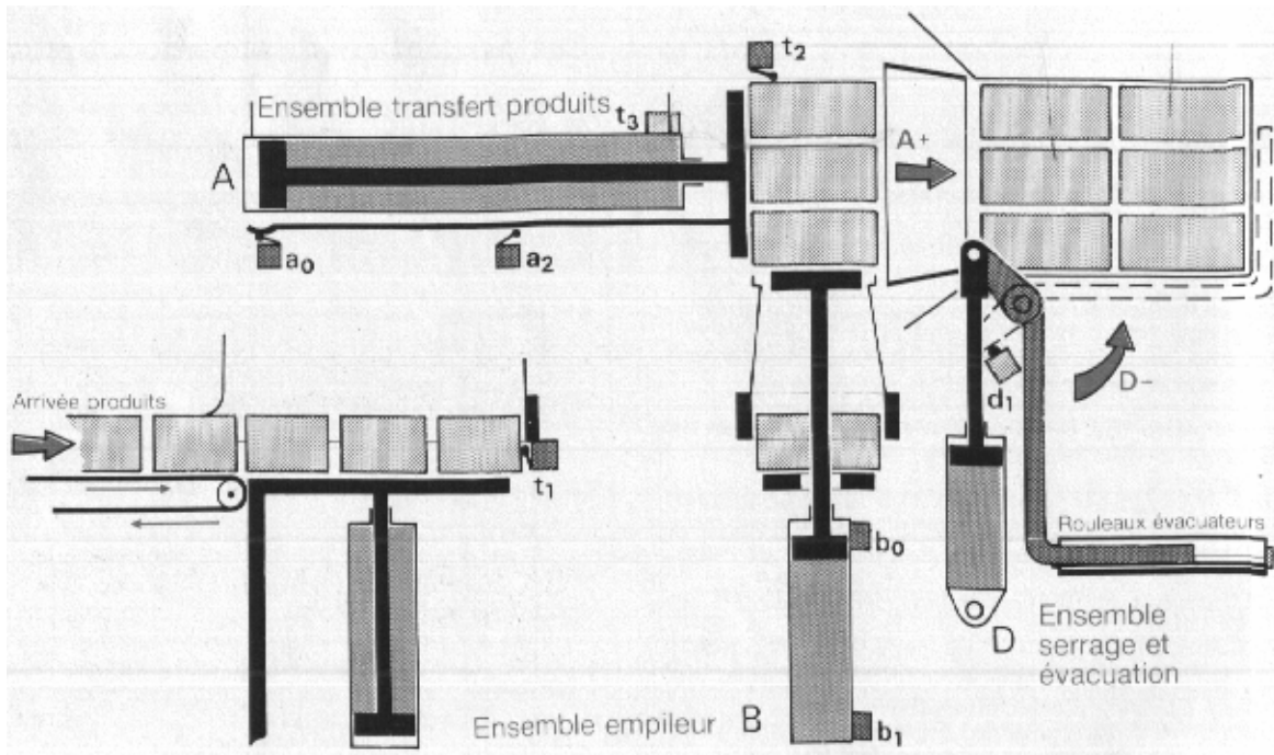
Figure 7 : Machine d'encaissage semi-automatique (vérins et capteurs montrés)
