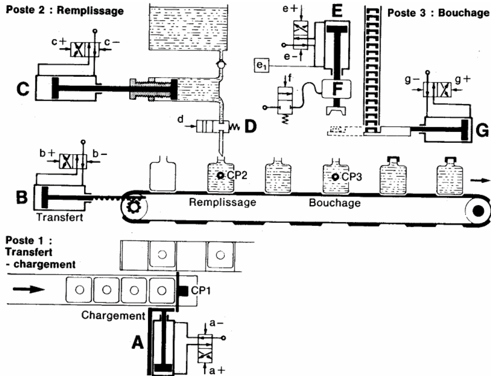
Figure 4 : Machine à remplir et à boucher
