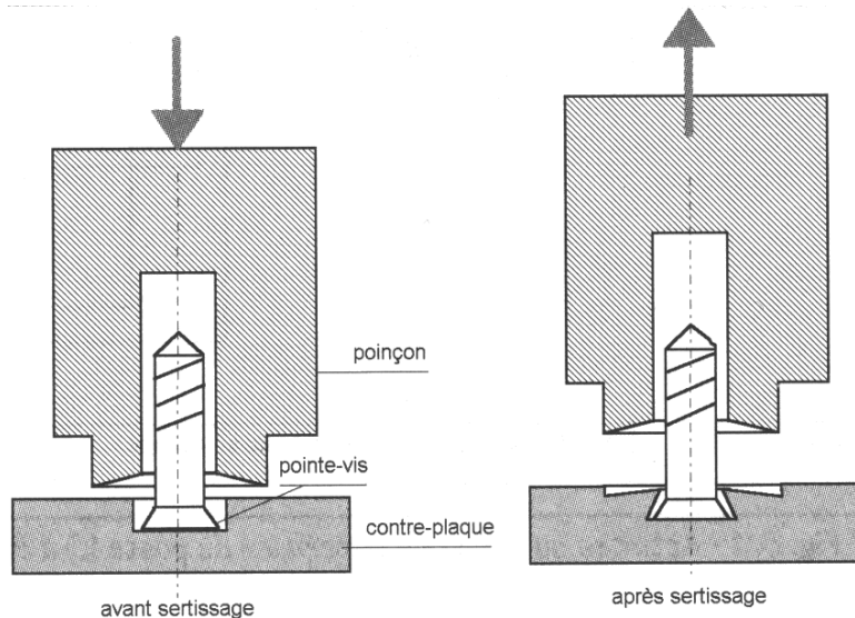
Figure 13 : Principe du sertissage
