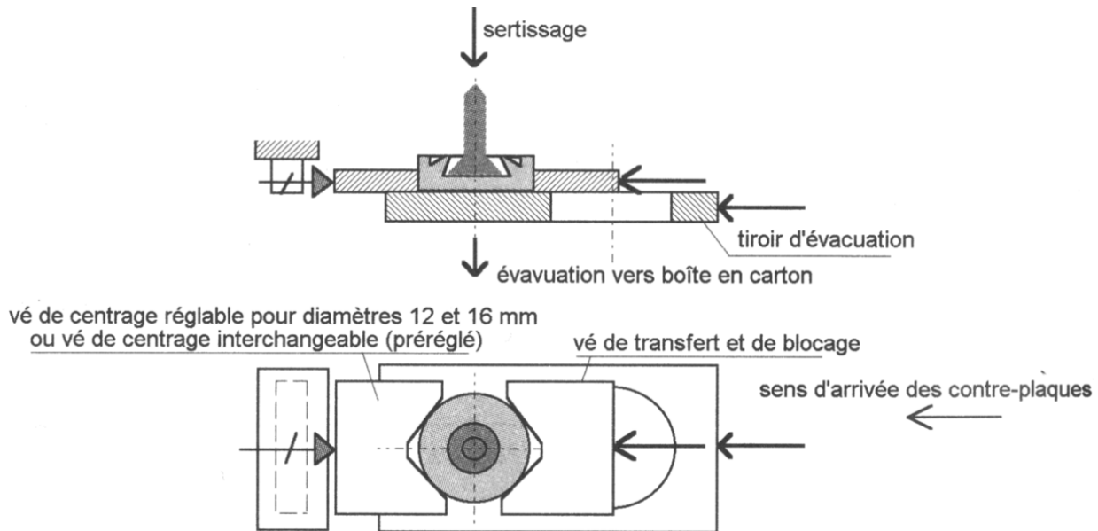
Figure 15 : Système de serrage et d'évacuation
