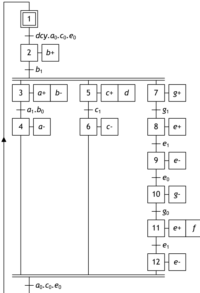
Figure 5 : GRAFCET du fonctionnement normal de la machine à remplir et à boucher
