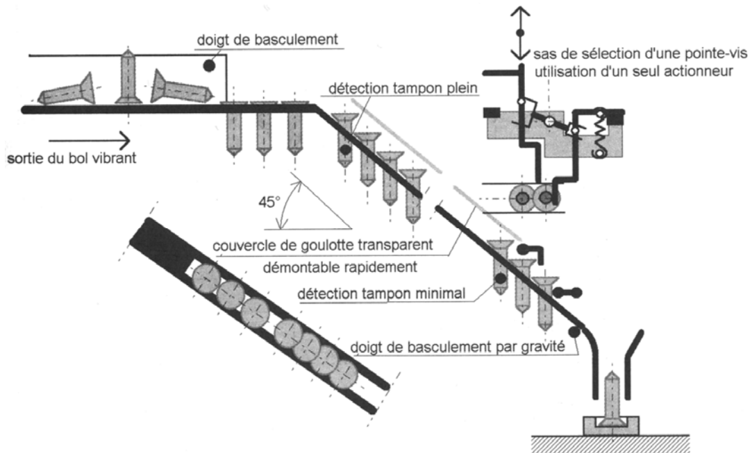
Figure 16 : Système d'acheminement de vis
