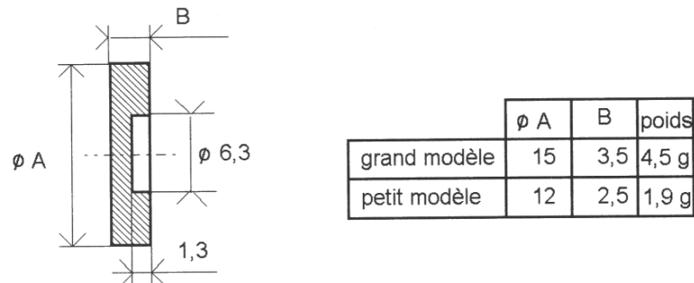
Figure 12 : Détail de la contreplaque
