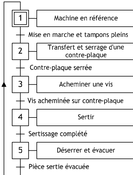
Figure 19 : GRAFCET de niveau 1 du fonctionnement normal du système de sertissage
