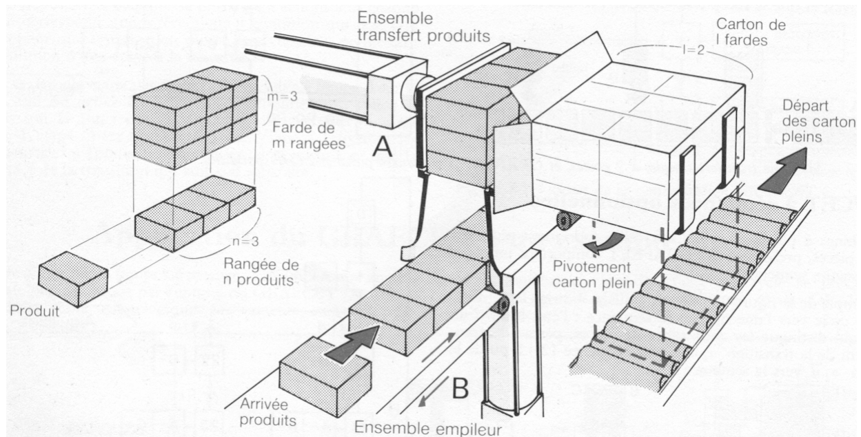
Figure 6 : Machine d'encaissage semi-automatique
