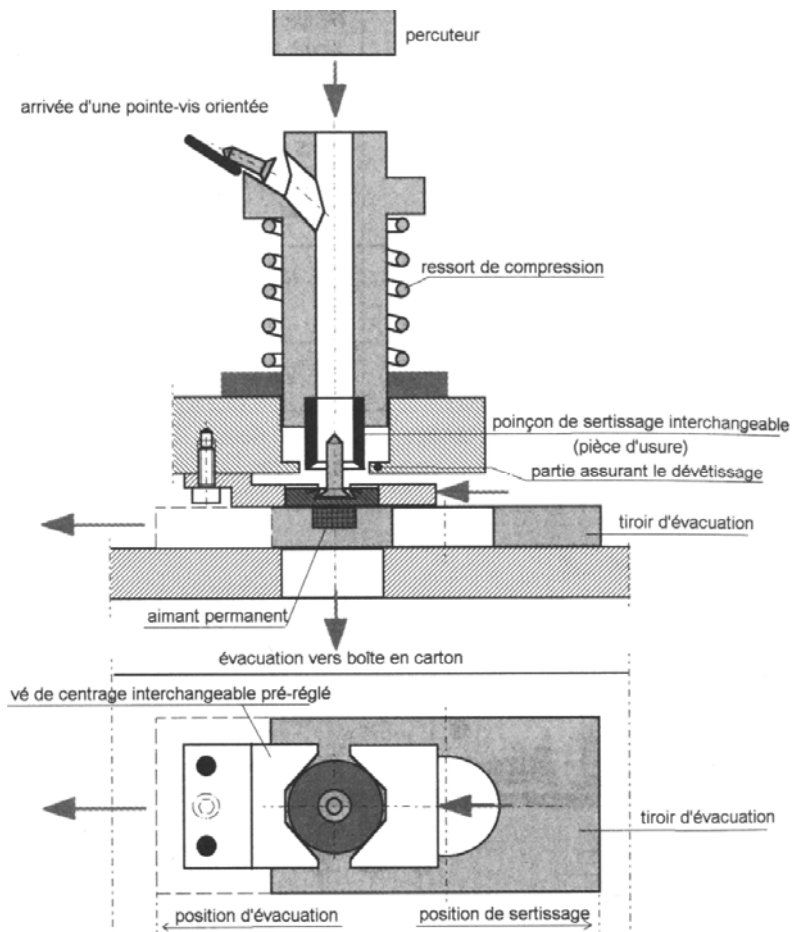
Figure 17 : Détail de l'acheminement des vis
