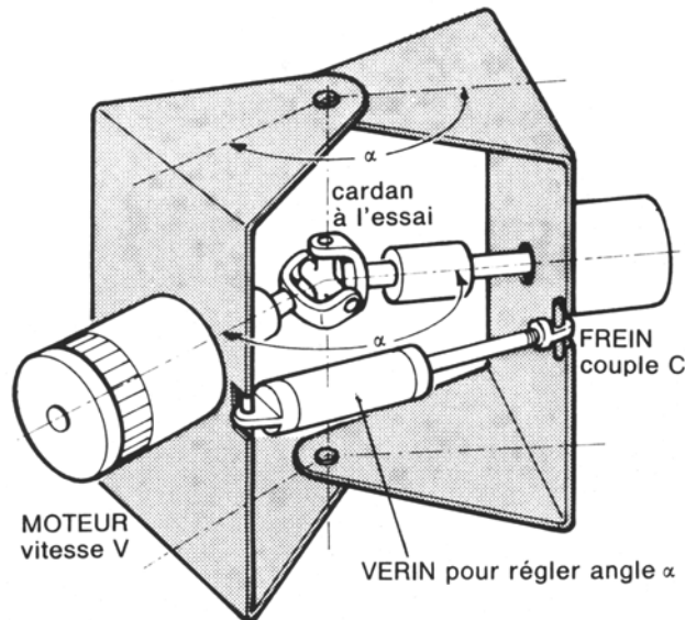
Figure 1 : Machine d'essai semi-automatique
