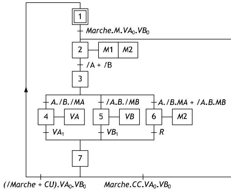
Figure 10 : GRAFCET du fonctionnement normal du système de tri automatique
